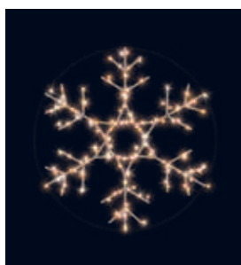
SNOW FLAKE 202013 Ø1 m. 6 Kg. 13 W.
